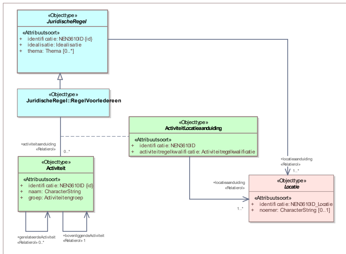
Figuur 31 Uitsnede uit IMOW-diagram voor objecttype Activiteit
