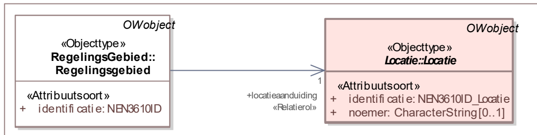
Figuur 43 Uitsnede uit IMOW-diagram voor objecttype Regelingsgebied
