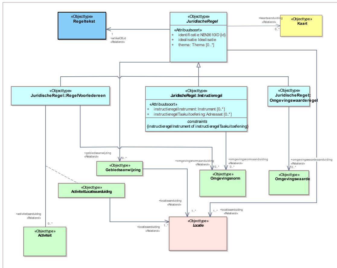
Figuur 22 Uitsnede uit IMOW-diagram voor objecttype Juridische regel
