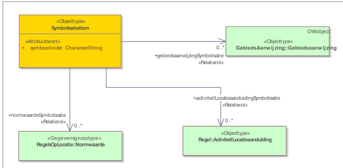
Figuur 40 Uitsnede uit IMOW-diagram voor objecttype SymbolisatieItem
