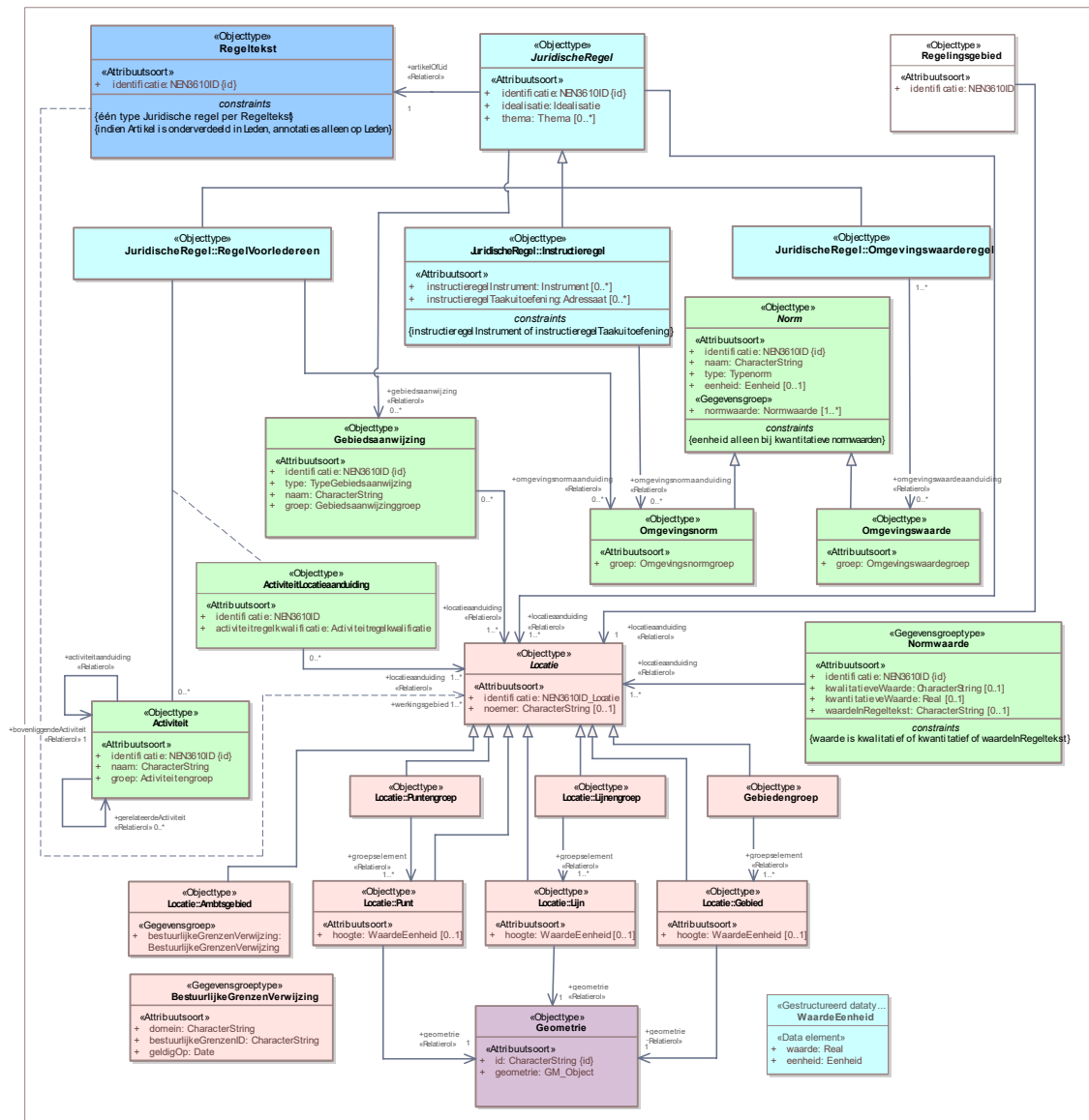
Figuur 20 IMOW-UML-klasediagram de AMvB/MR
