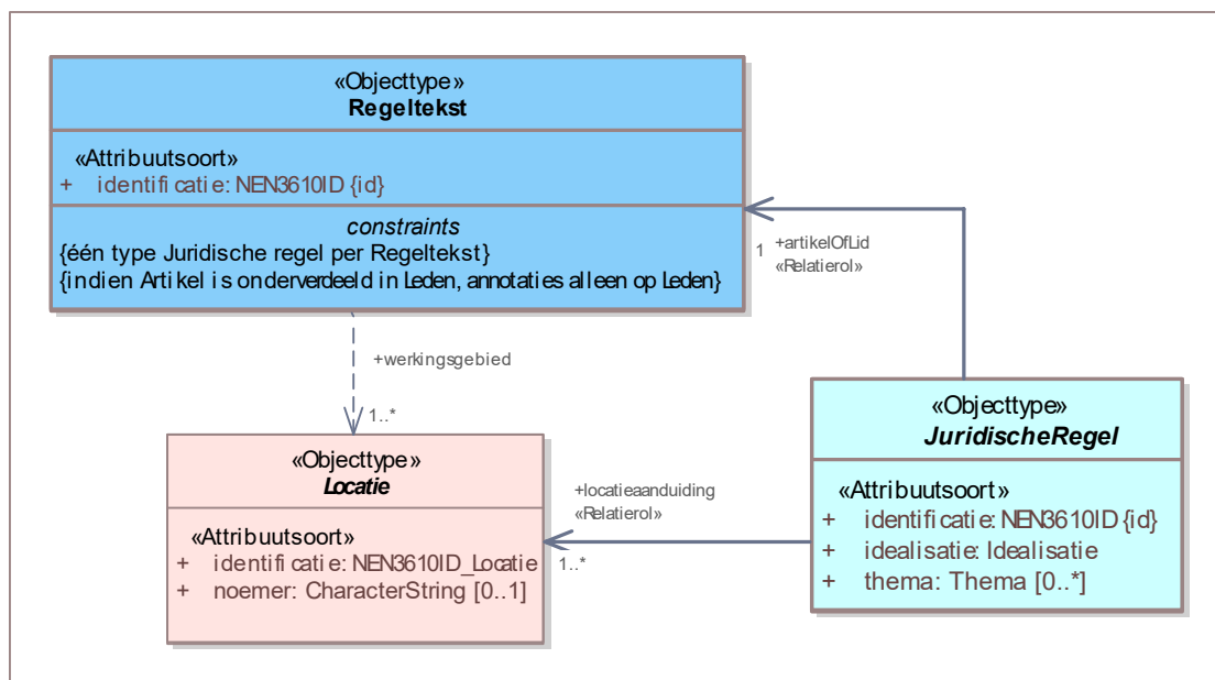
Figuur 21 Uitsnede uit IMOW-diagram voor objecttype Regeltekst
