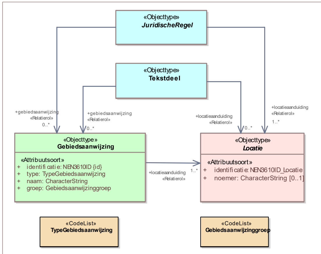
Figuur 38 Uitsnede uit IMOW-diagram voor objecttype Gebiedsaanwijzing
